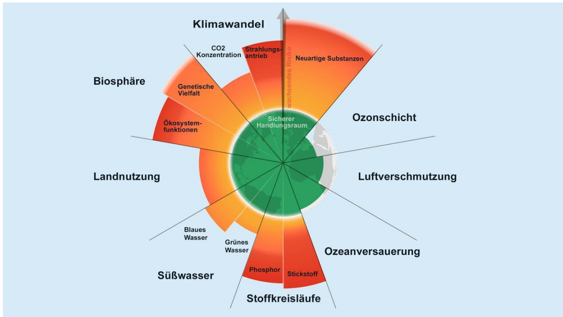
Grafik: Deutschlandfunk, ursprünglich von Azote für das Stockholm Resilience Centre auf Basis von der Analyse in Richardson et al 2023
